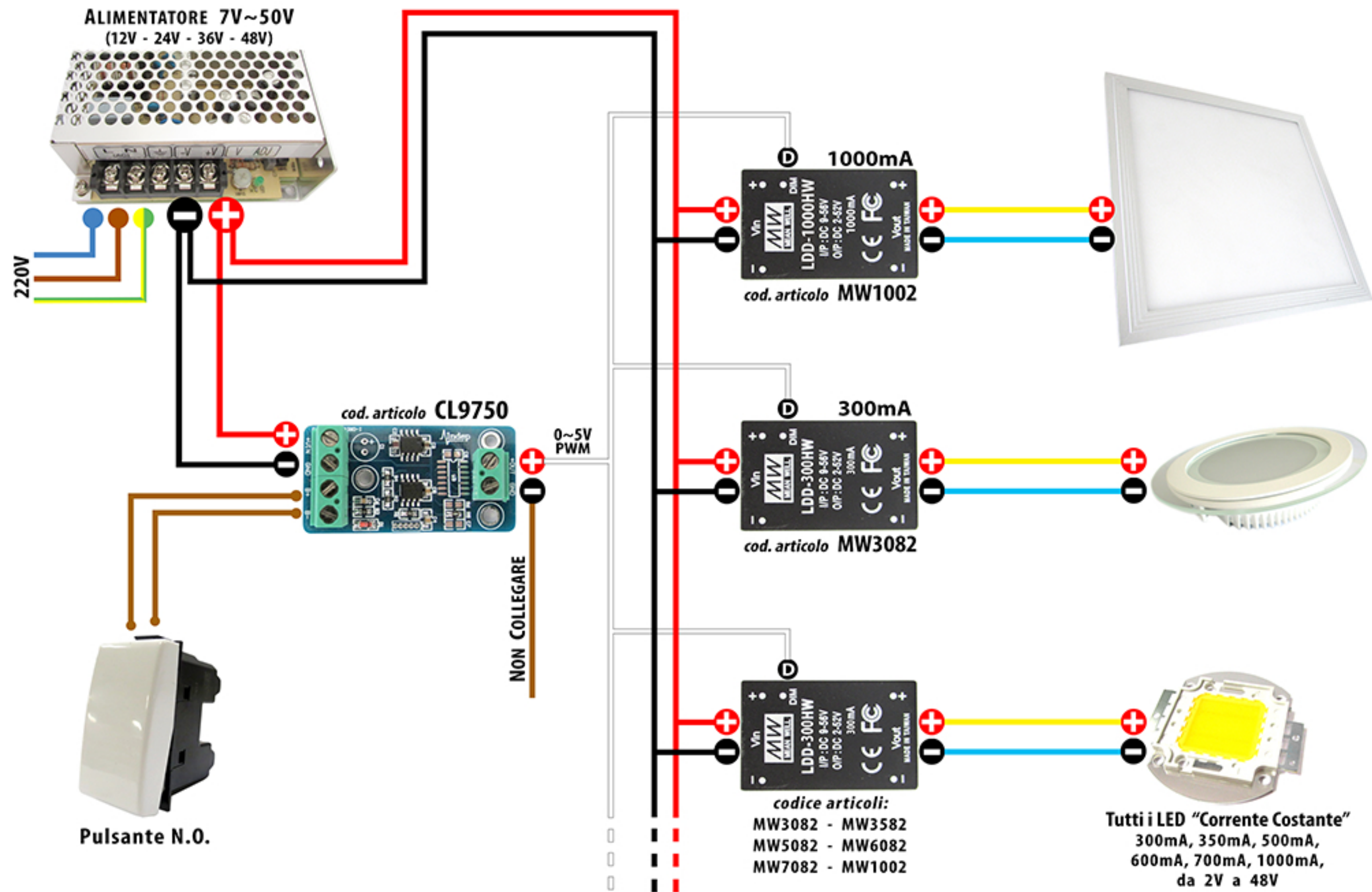
SCHEMA ELETTRICO - INSTALLAZIONE CON UNICO ALIMENTATORE
