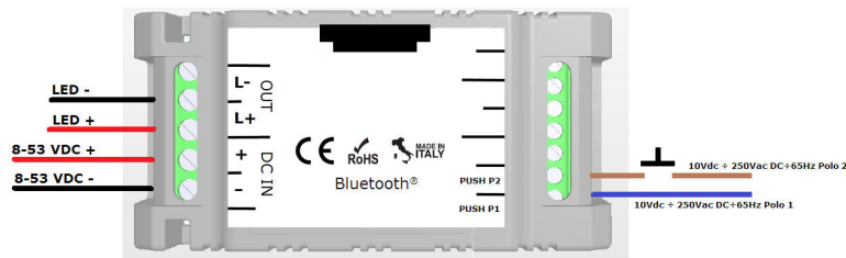
COLLEGAMENTO BLE L400MC04T1A01 - FIGURA N. 6
